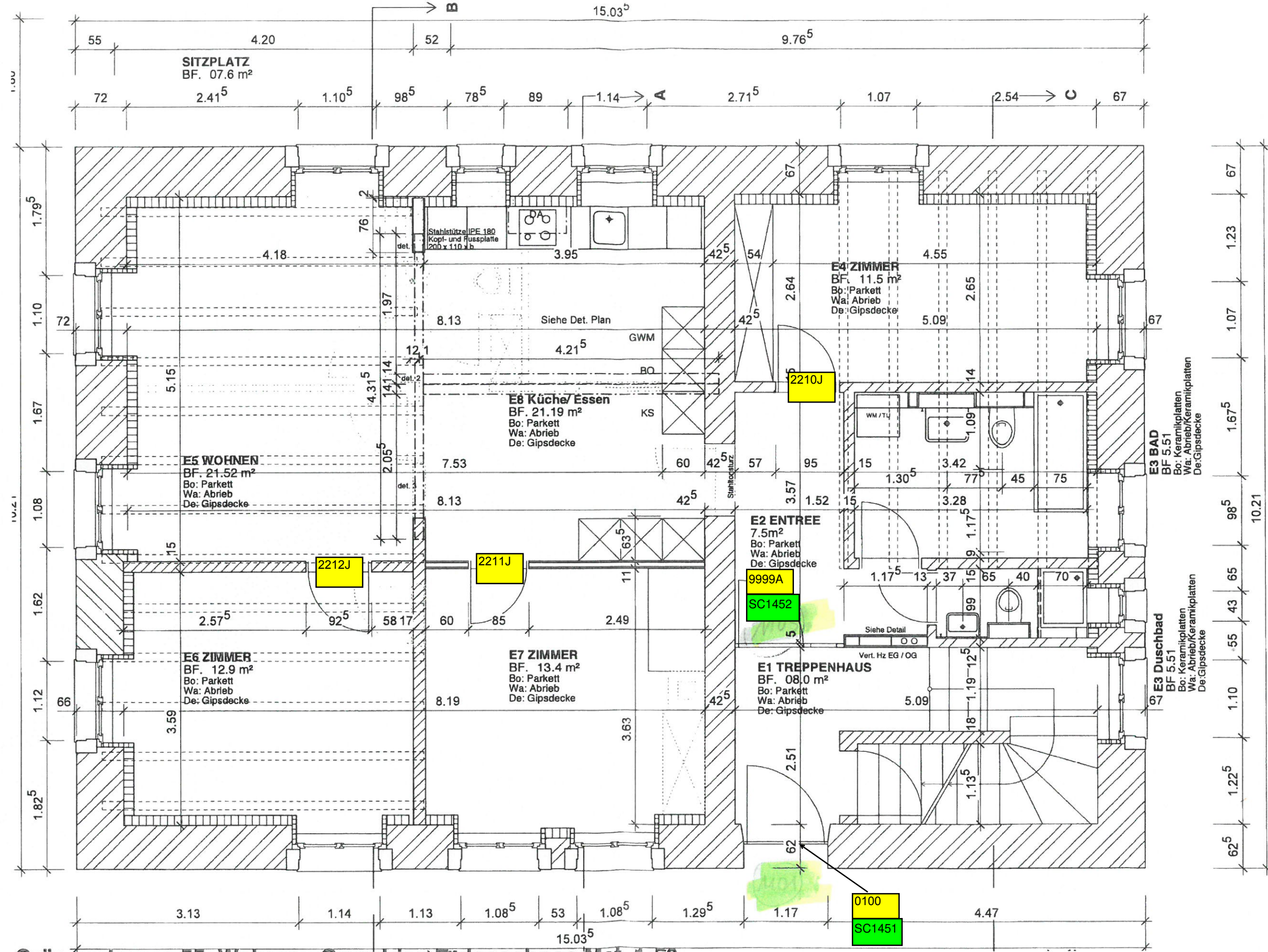
Grünaustrasse 55, Wabern - Grundriss Erdgeschoss Mst. 1:50
